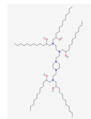
CAS Number: 1220890-25-4
